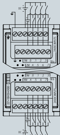
SM 1221 DI 16 x 24 V DC
