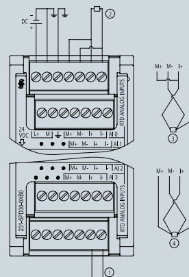
① 短接未使用的 RTD 输入 ③ 3 线制 RTD ② 2 线制 RTD ④ 4 线制 RTD
