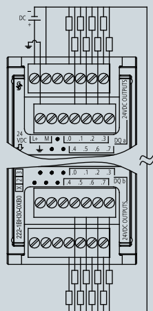
SM 1222 DQ 16 x 24 V DC
