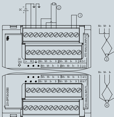
① 短接未使用的 RTD 输入 ③ 3 线制 RTD ② 2 线制 RTD ④ 4 线制 RTD
